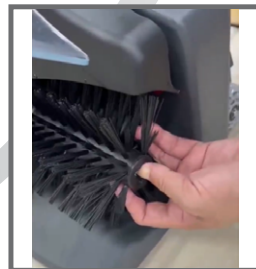
快拆式滾刷設計
