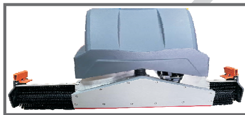
清洗滾刷拆裝卡扣設計
